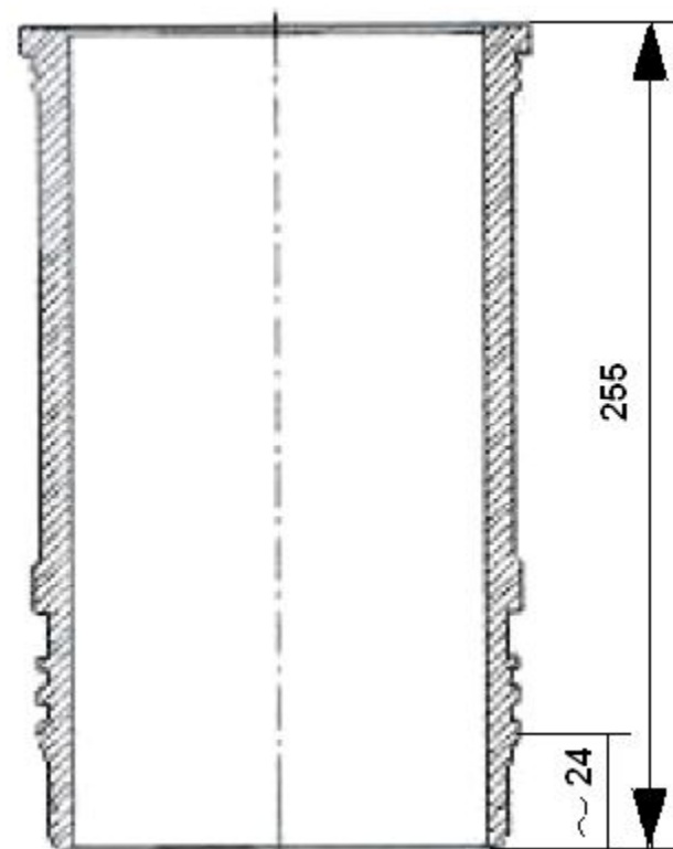
Рис. 2 Гильза цилиндров 7511.1002021-01. Производства ЗАО «Костромской завод автокомпонентов» или производства ООО «Мотордеталь-Конотоп»
