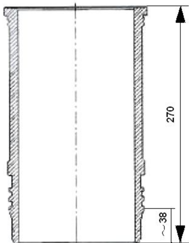
Рис. 1 Гильза цилиндров 7511.1002021-01. Производства ОАО «Автодизель»
