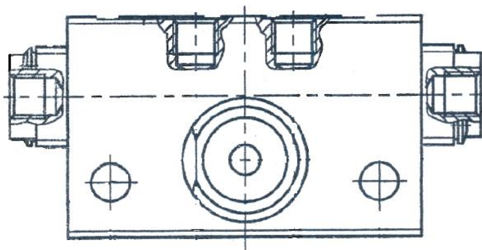
Рис. 2. Воздухораспределитель 358-033CO2 (8.9076) производства фирмы «Камоцци Пневматика»
