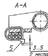
Рисунок 1. Установка воздухораспределителя фирмы ООО «Камоцци Пневматика» на коробки передач с серийными воздухопроводами.
