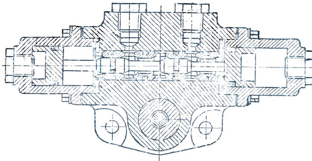
Рис. 3. Воздухораспределитель 238H-1723009-01 производства ОАО «Автодизель»
