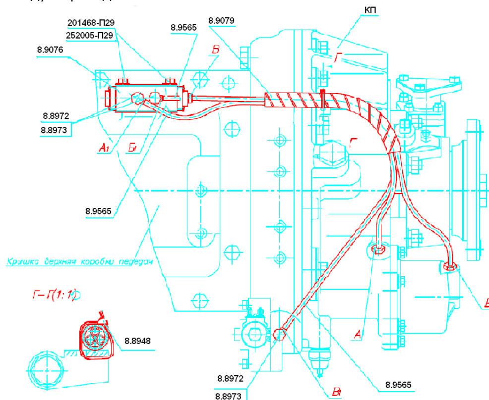
Рис.1. Установка воздухораспределителя и воздухопроводов производства ООО «Камоцци Пневматика».
